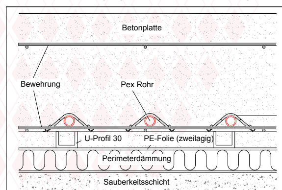
Beispiel: Rohrbefestigung auf der unteren Bewehrung
